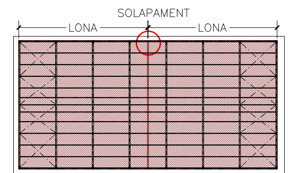
PLANTA COBERTA LONA Esc. 1/600
