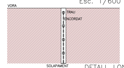
DETALL LONA (planta) SOLAPAMENT E. 1/2.5
