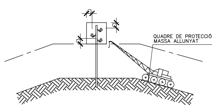
PAS PER SOTA DE LÍNIES AÈRIES DE BAIXA TENSÍO
